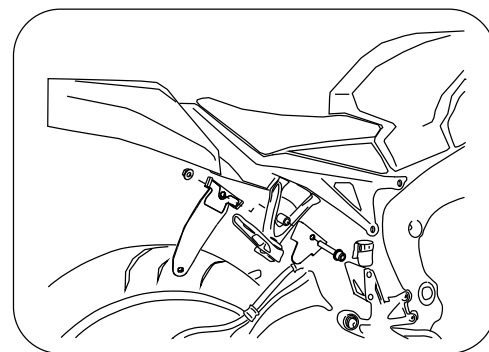
図3.サイレンサーステー取り付け
