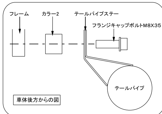
図2.テールパイプステー取り付け
