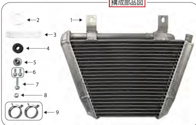
構成部品図
