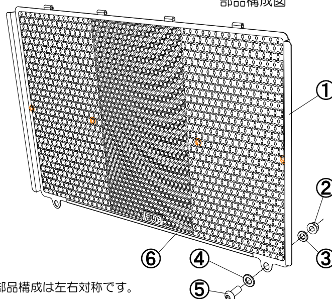
部品構成図
