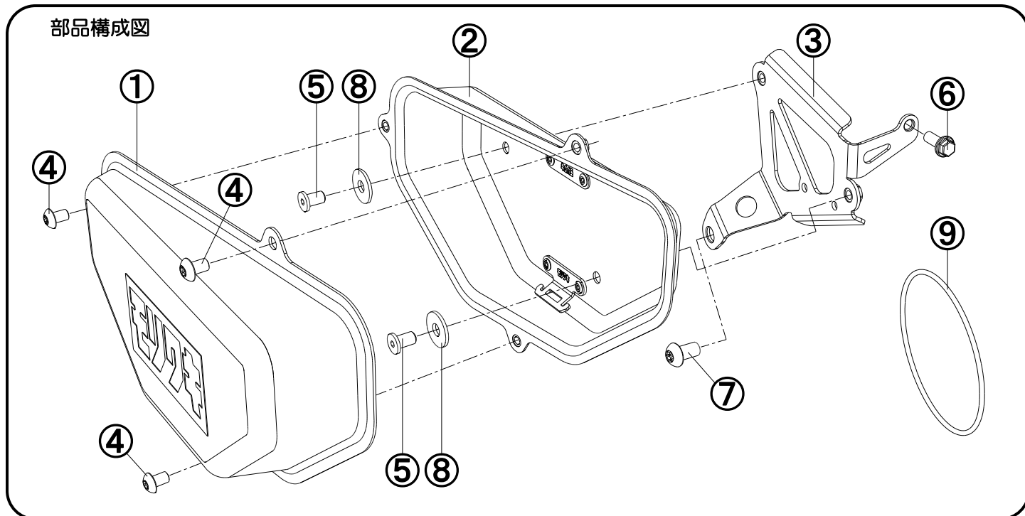
【構成部品表】
